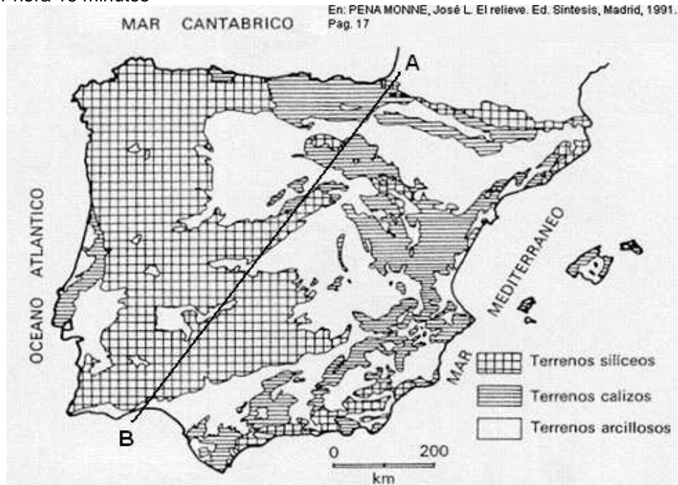
Doc. 1 Mapa litológico de la Península Ibérica
