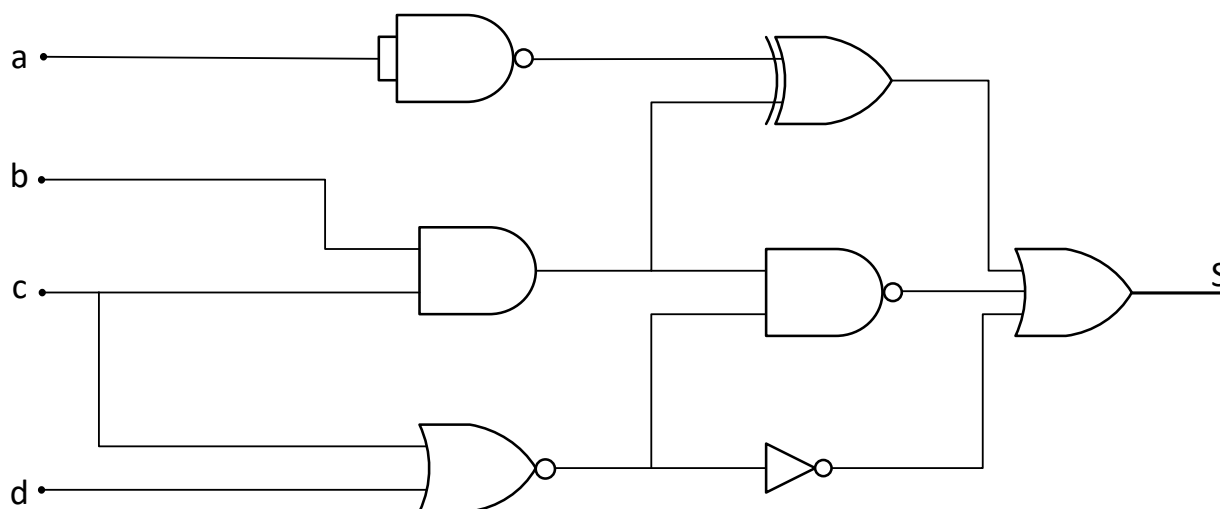
Figura 3. Circuito lógico.
